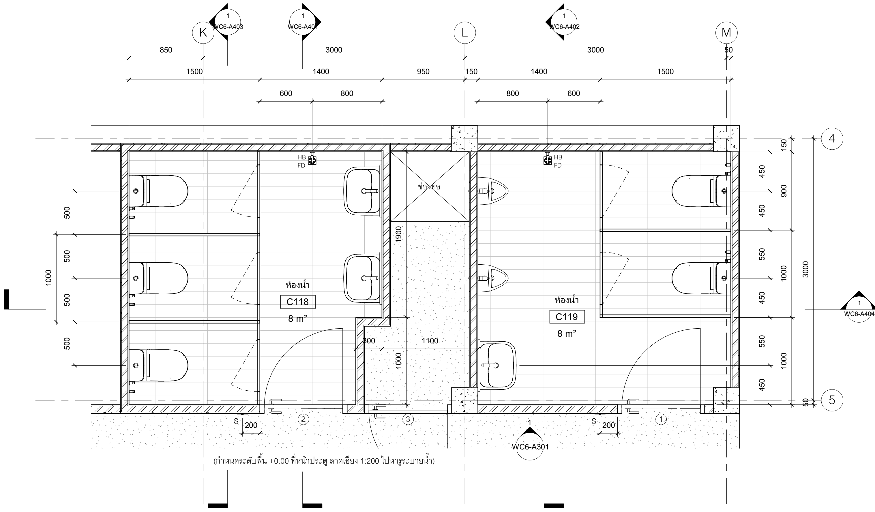
1 แปลนพื้นที่ห้องน้ำ C118 & C119, ห้องน้ำ C214 & C215, ห้องน้ำ C313 & C314 1:25
