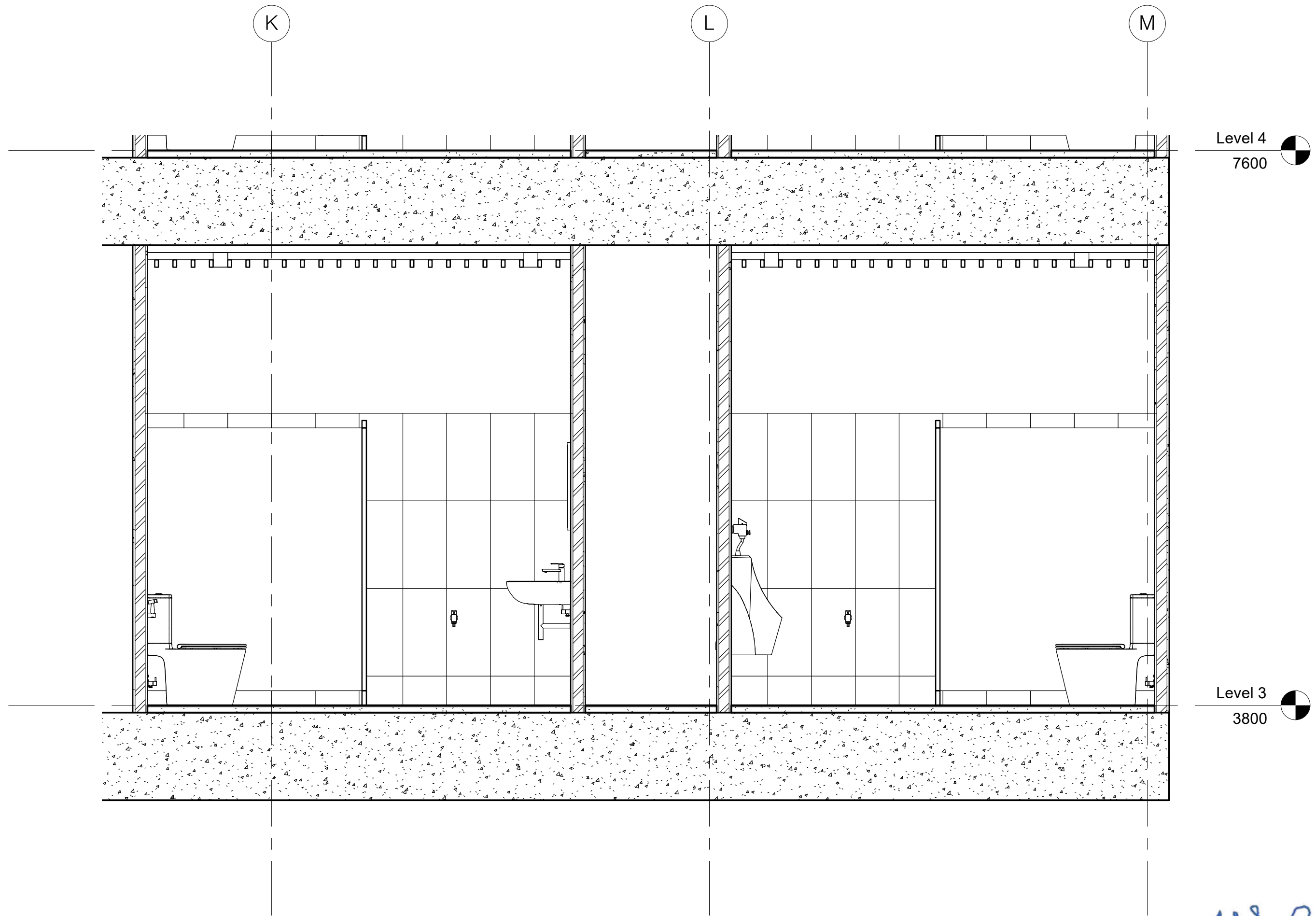
1 รูปตัด WC6 - 4 1 : 25
