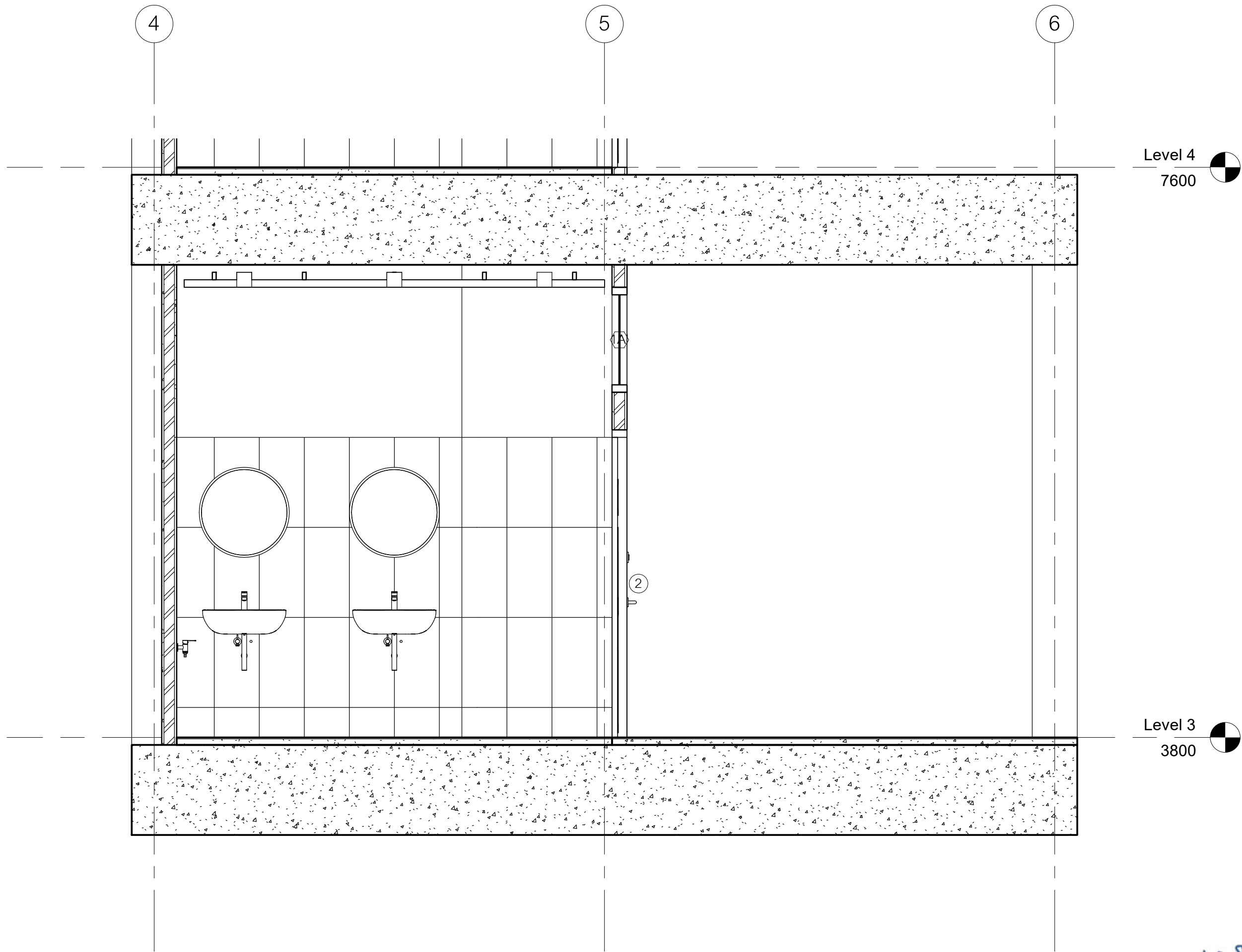
1 รูปตัด WC6 - 1 1 : 25
