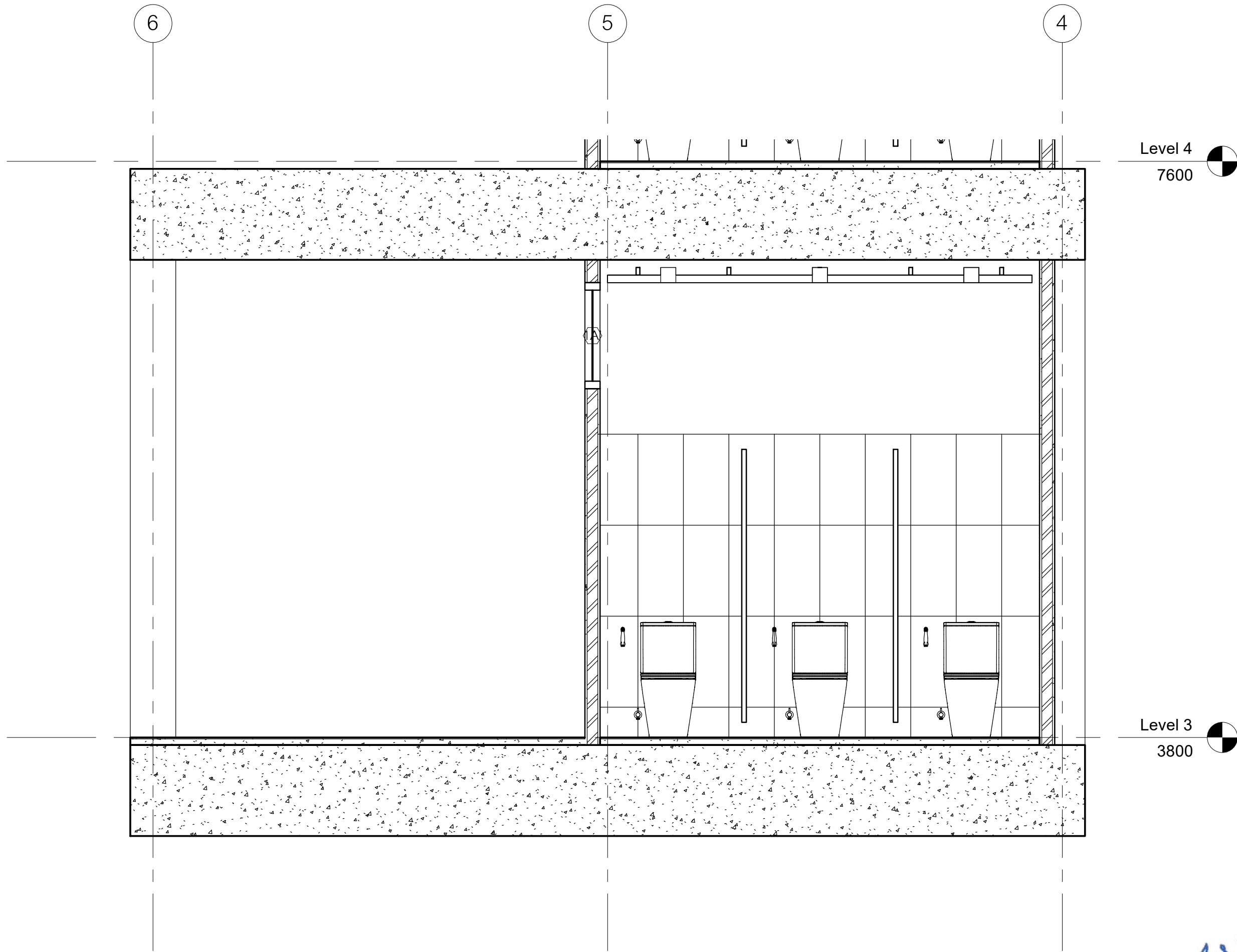
1 รูปตัด WC6 - 3 1 : 25
