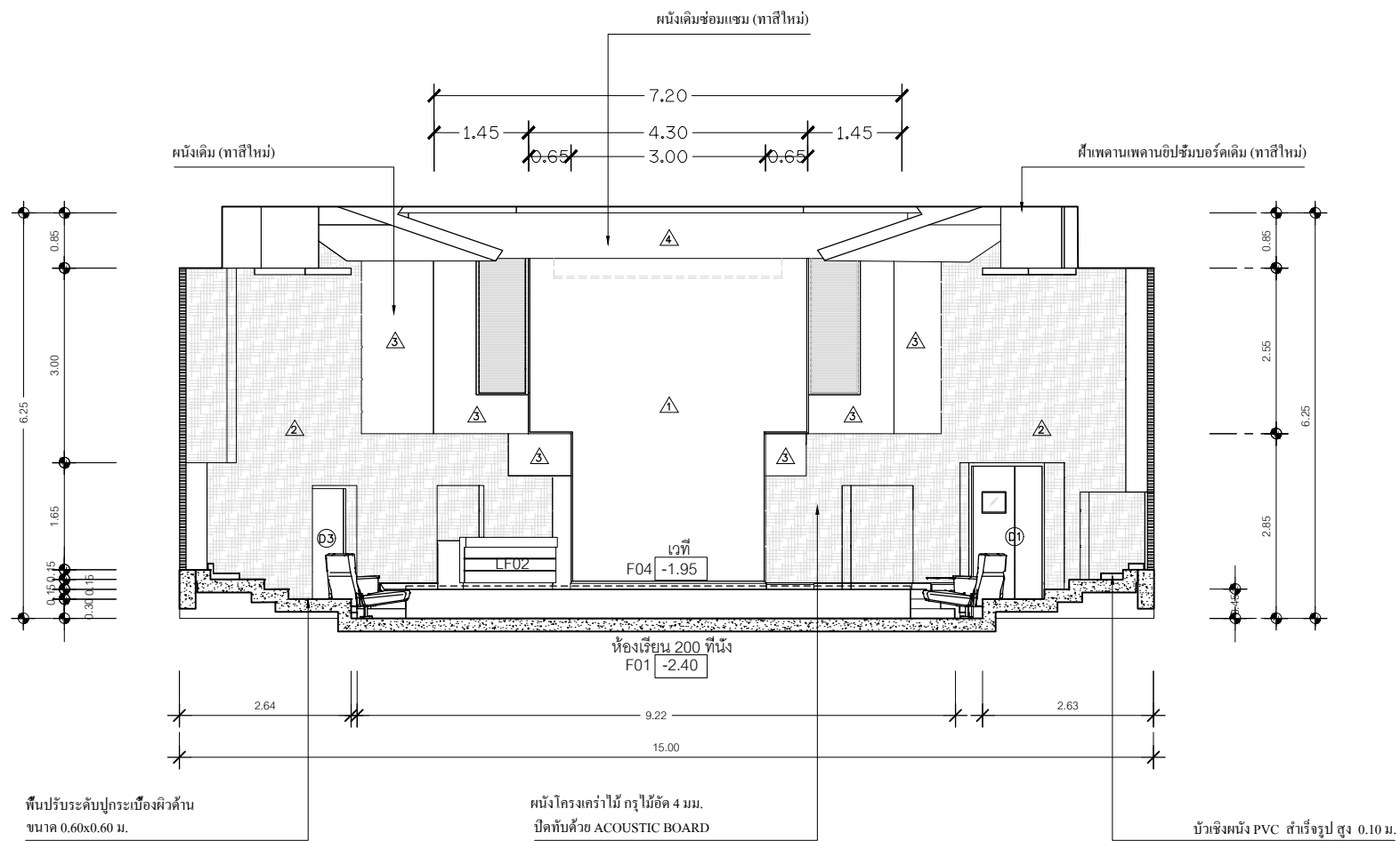
แปลนห้องเรียน 3301 (รูปตัด D) SCALE1:100
