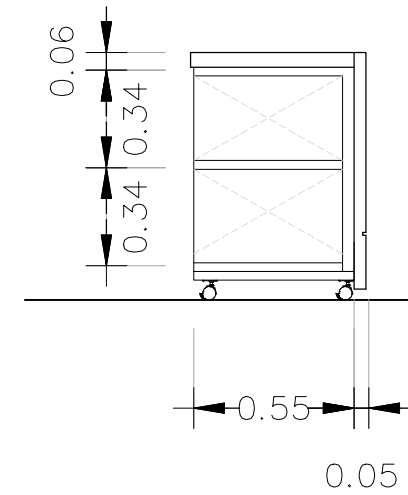
รูปตัด B
