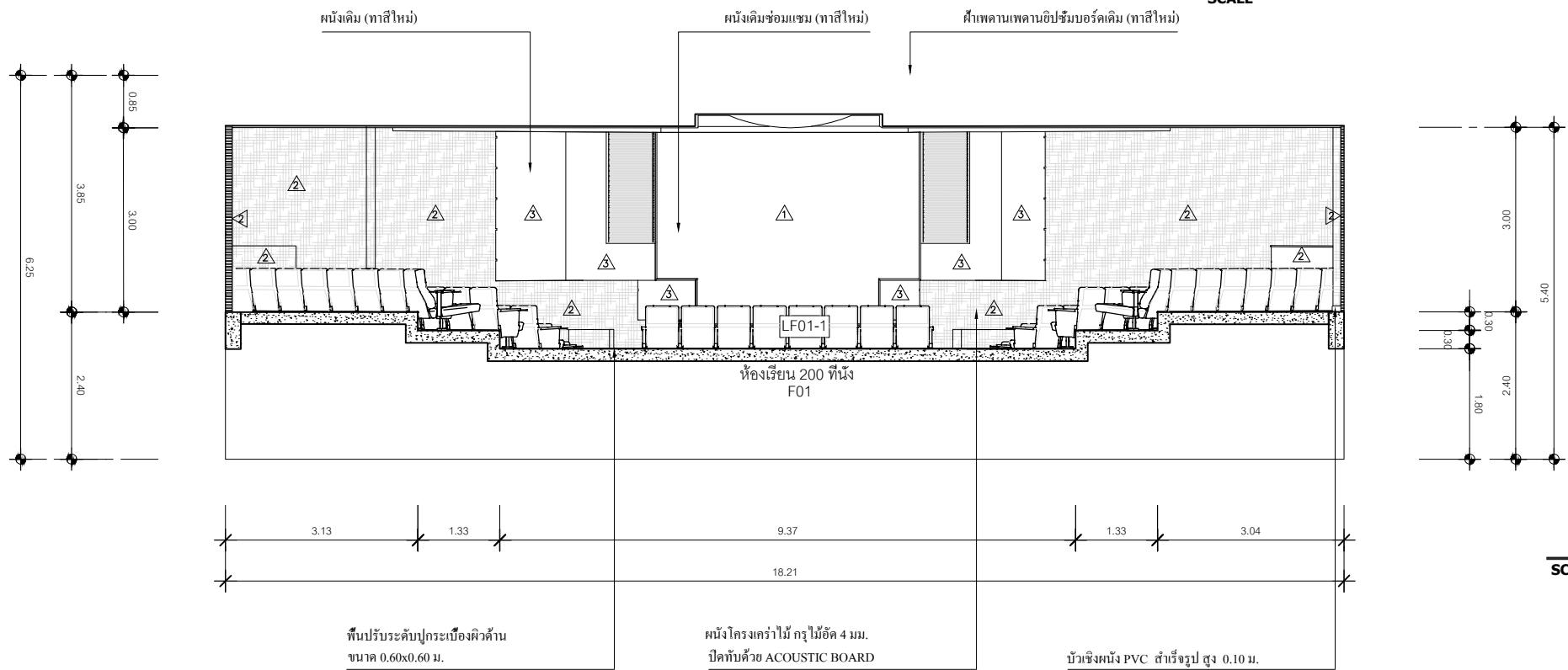
แปลนห้องเรียน 3301 (รูปตัด C) SCALE 1:100
