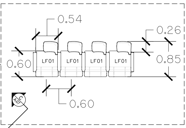
แบบขยายระยะเก้าอี้ SCALE 1:50
