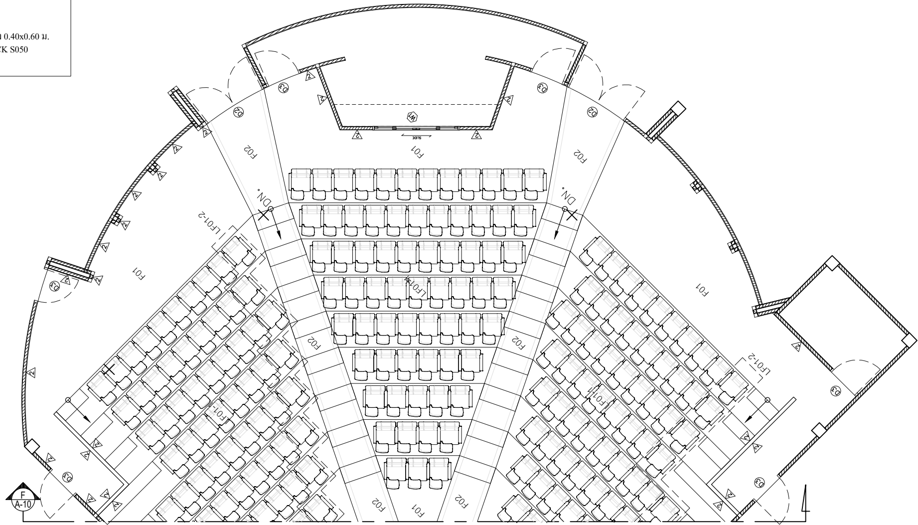
แปลนห้องเรียน 3301 (รูปตัด F) SCALE 1:100
